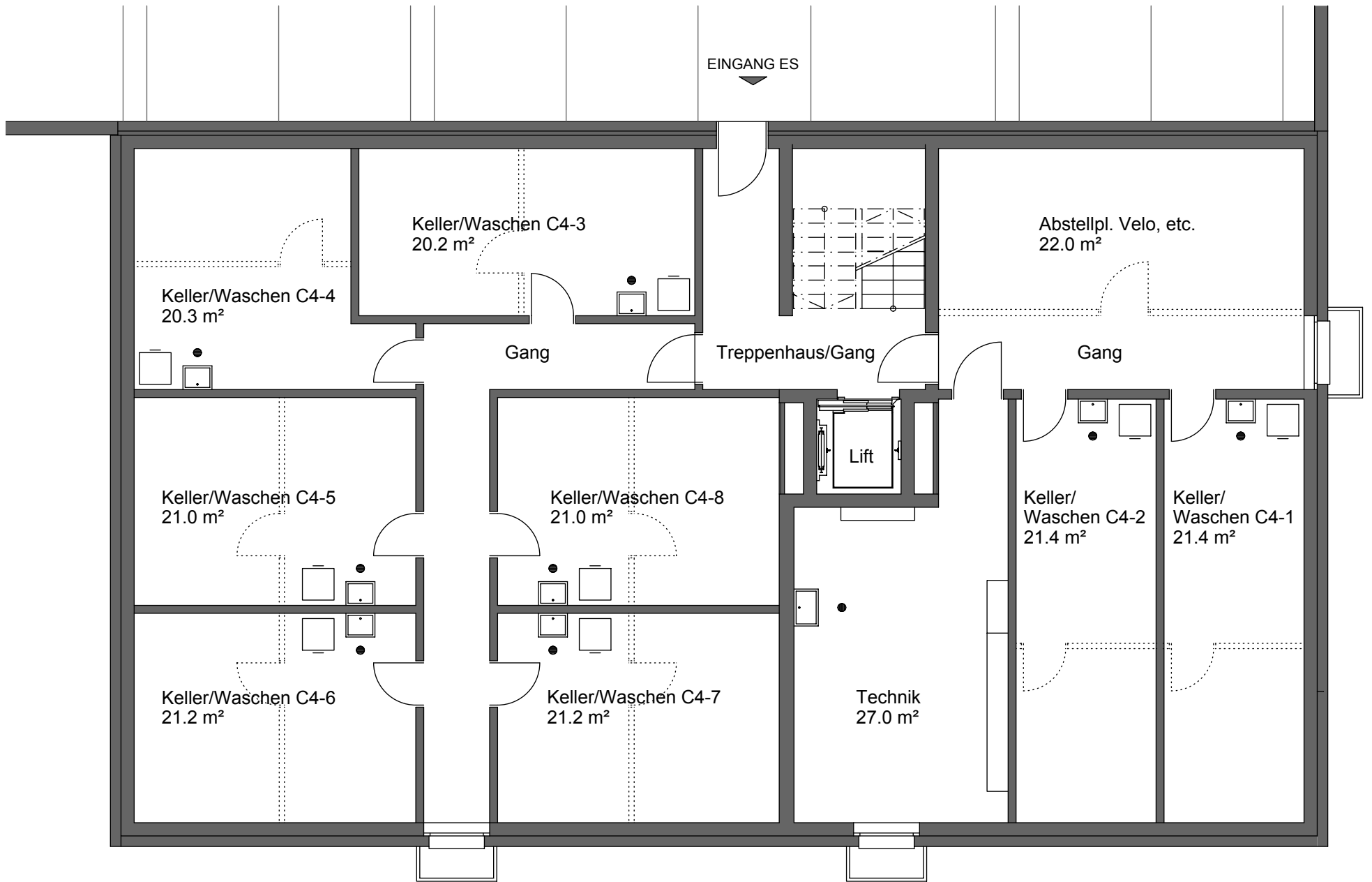
MFH Chappelbode 4, Escholzmatt Untergeschoss 1:100
